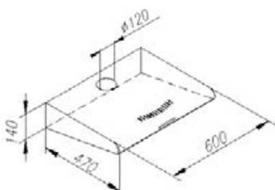
Montageabstand über Kochfeld Elektro 450 mm, Gas 650 mm
