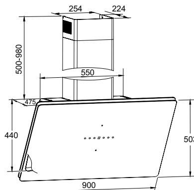
Montageabstand über Kochfeld Elektro 450 mm, Gas 650 mm
