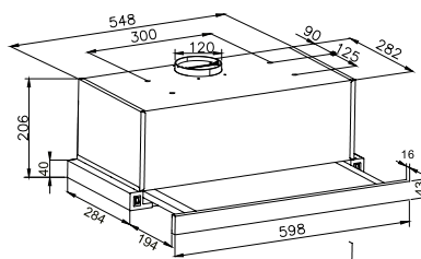
Montageabstand über Kochfeld Elektro 450 mm, Gas 650 mm
