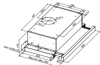
Montageabstand über Kochfeld Elektro 450 mm, Gas 650 mm
