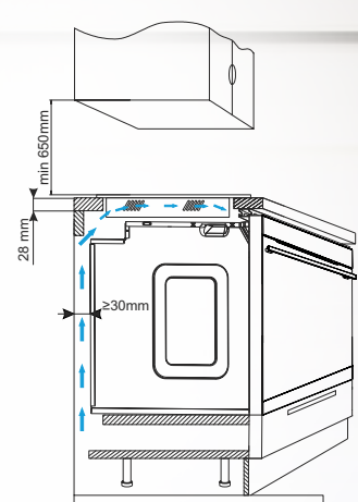
Einbau über einem Backofen
