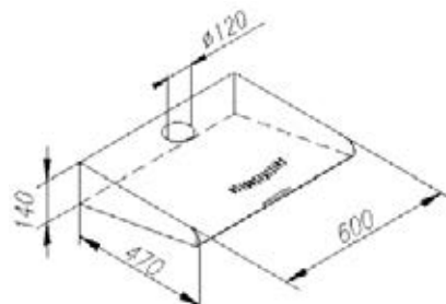
Montageabstand über Kochfeld Elektro 450 mm, Gas 650 mm
