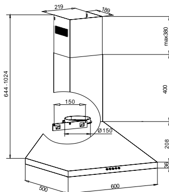
Montageabstand über Kochfeld Elektro 450 mm, Gas 550 mm
