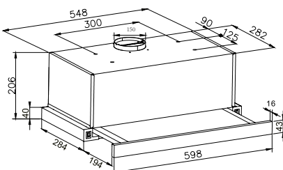
Montageabstand über Kochfeld Elektro 450 mm, Gas 650 mm
