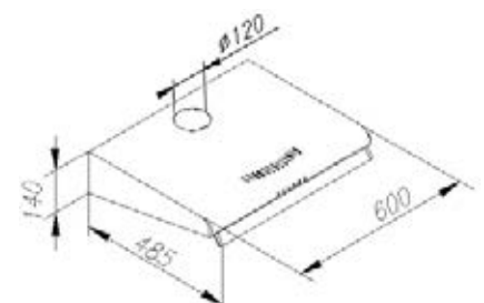
Montageabstand über Kochfeld Elektro 450 mm, Gas 650 mm
