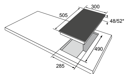
*Abmessungen inkl. Verbindungsbox
