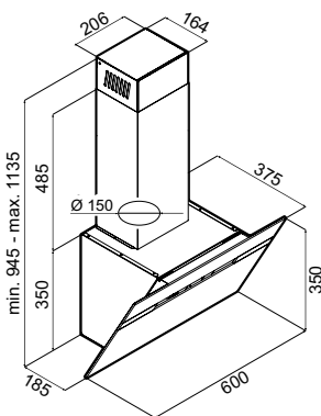
Montageabstand über Kochfeld Elektro 450 mm, Gas 650 mm
