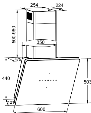
Montageabstand über Kochfeld Elektro 450 mm, Gas 650 mm
