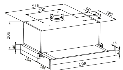
Montageabstand über Kochfeld Elektro 450 mm, Gas 650 mm
