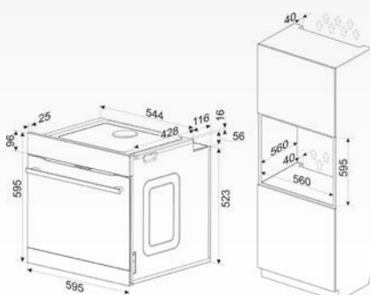
Montage ohne Lüftungsspalt vorne
