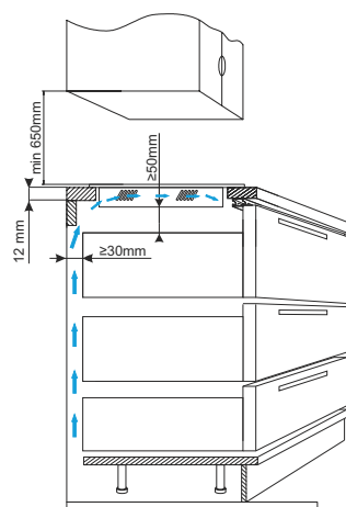
Einbau über einer Schublade
