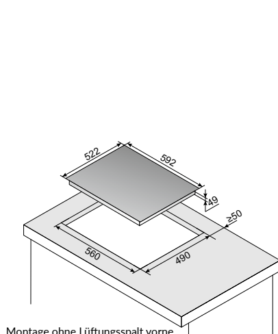
Montage ohne Lüftungsspalt vorne
