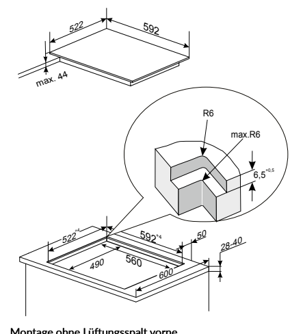
Montage ohne Lüftungsspalt vorne
