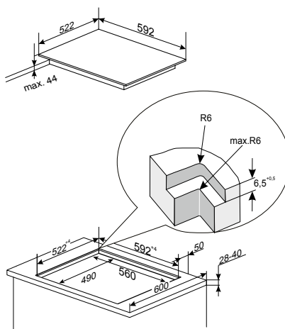
Montage ohne Lüftungsspalt vorne
