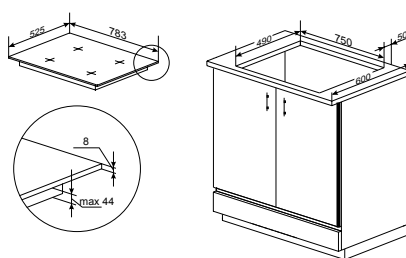
Montage ohne Lüftungsspalt vorne
